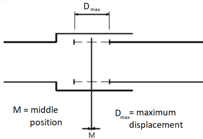
3. attēls. Sliežu ceļa kompensatora principālā shēma
