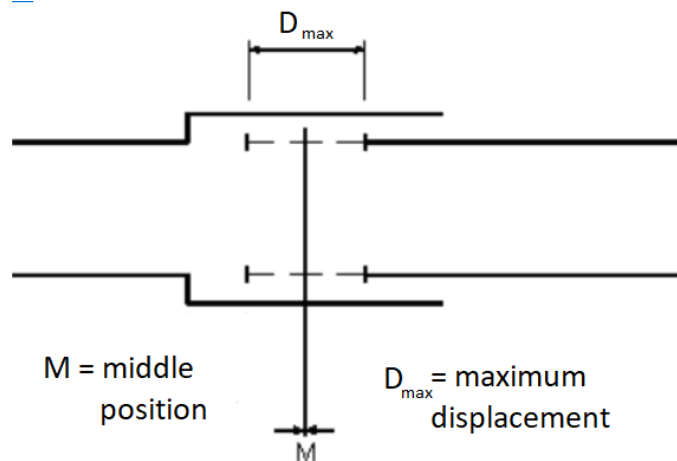
3. attēls. Sliežu ceļa kompensatora principālā shēma
