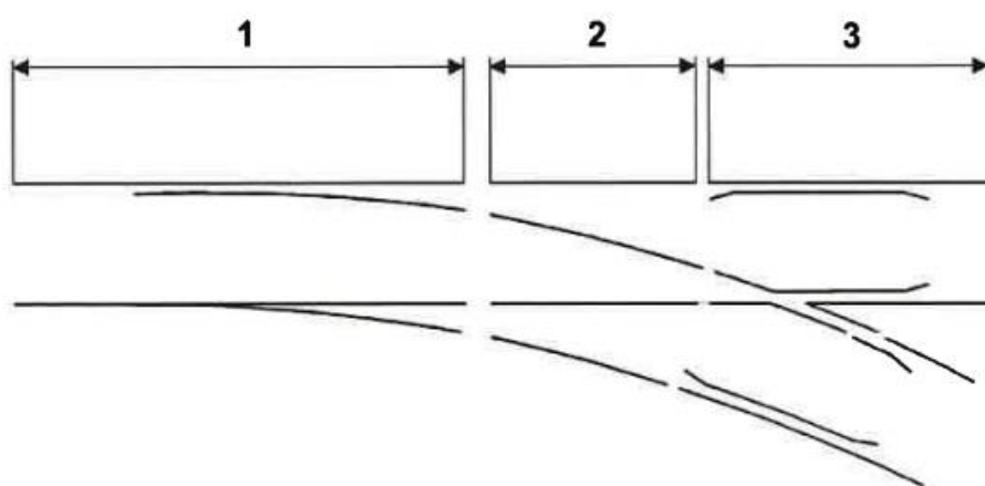
1 pav., Iešmo principinė schema
