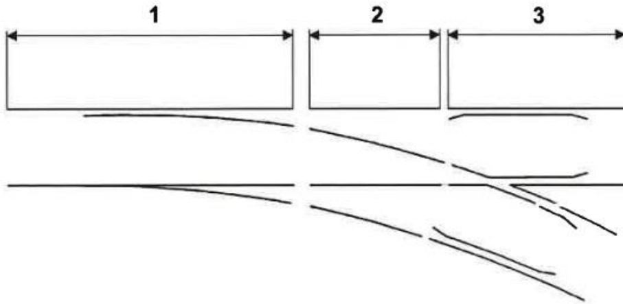
2 pav., iešmo principinė schema
